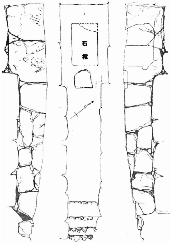
艸墓古墳石室 石室実測図
