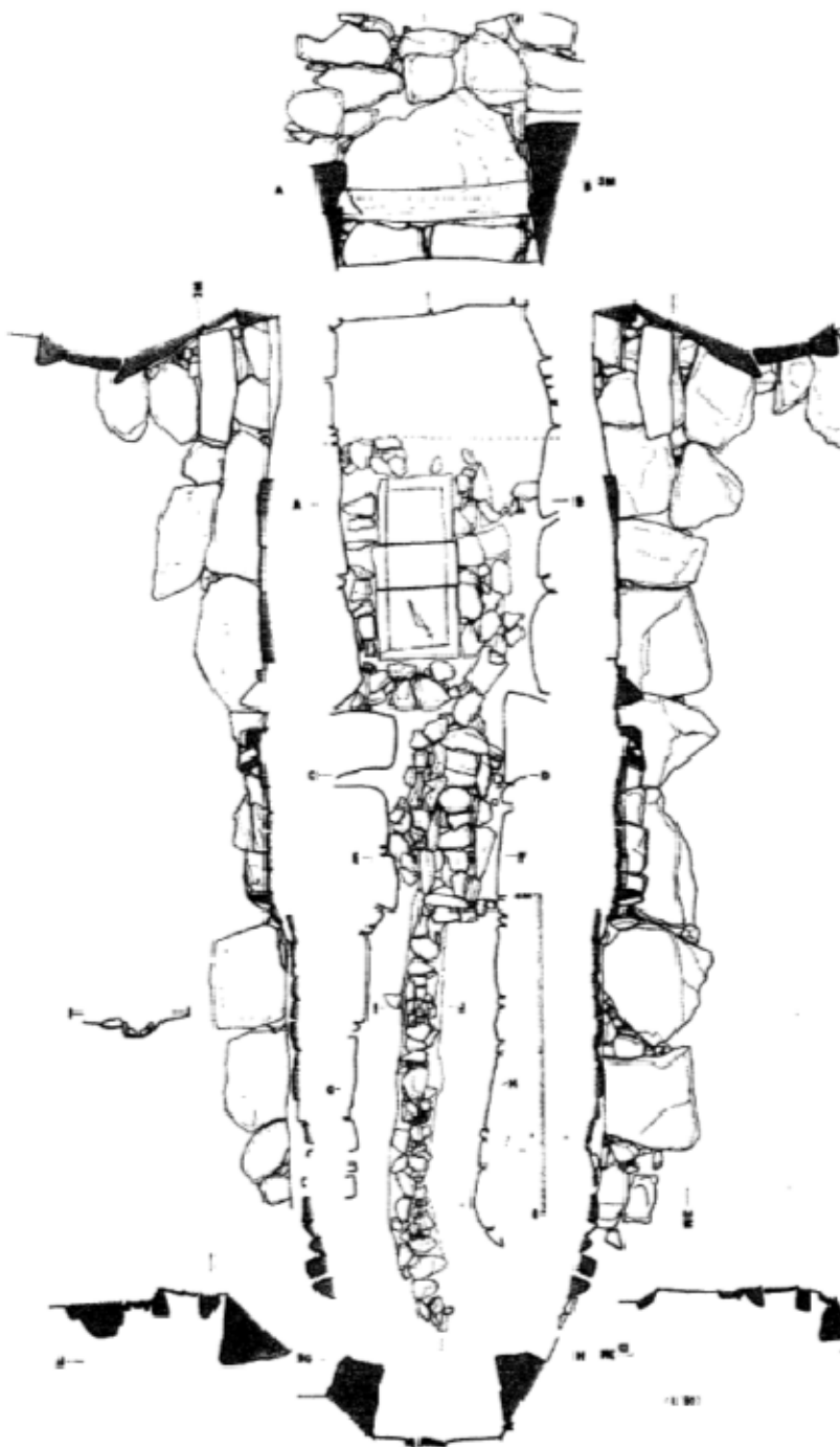
三里古墳石室実測図
